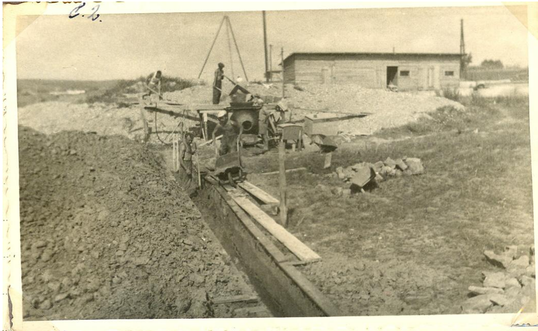
Kopání základů pro mateřskou školu – 16.8.1947
